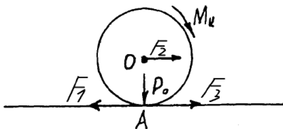
Рис. 2.1. Силы действующие на колесную пару
