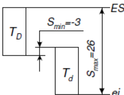
Рис. 2. Схема посадки.
