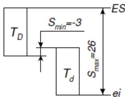
Рис. 2. Схема посадки.
